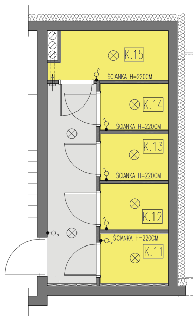
RZUT POMIESZCZEŃ
