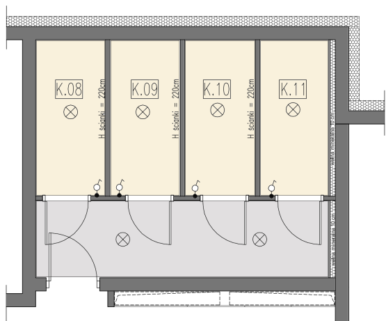
RZUT POMIESZCZEŃ
