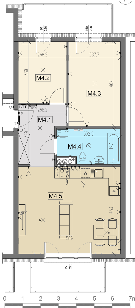
RZUT MIESZKANIA
