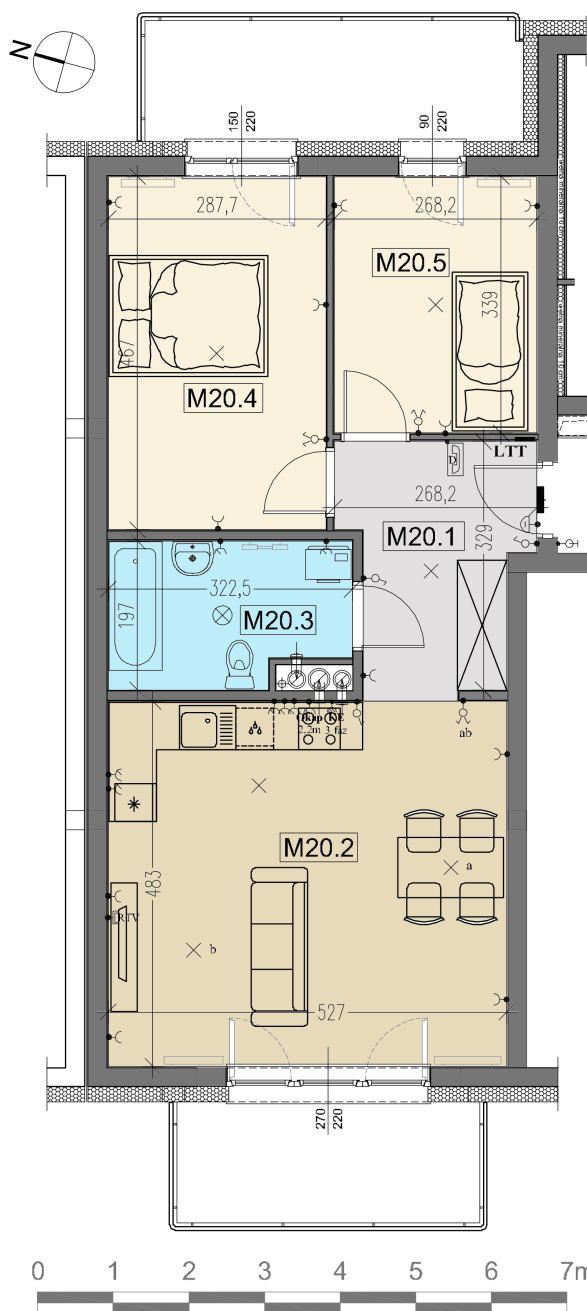
RZUT MIESZKANIA
