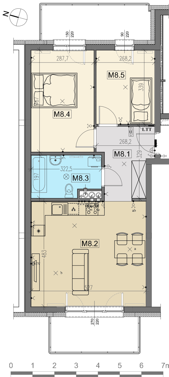
RZUT MIESZKANIA
