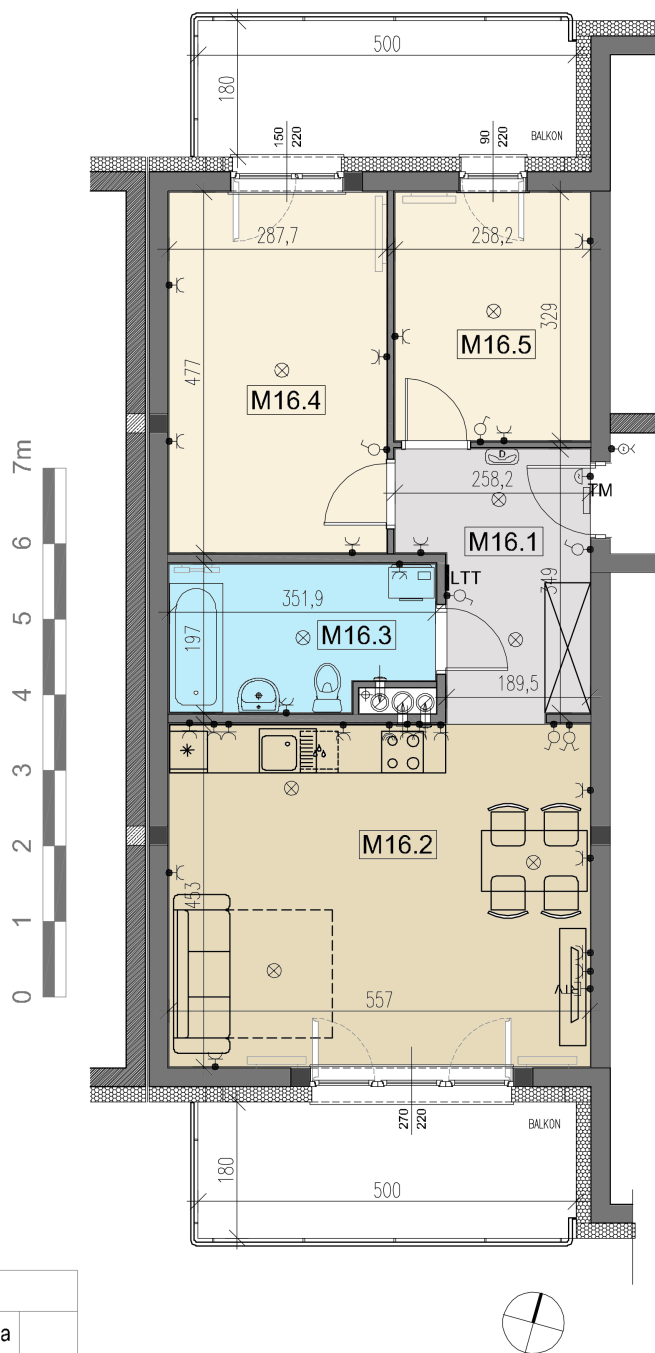
RZUT MIESZKANIA
