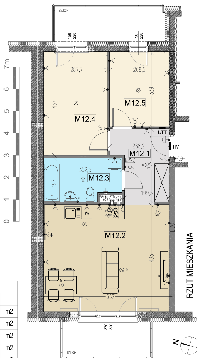
PLAN BUDYNKU
