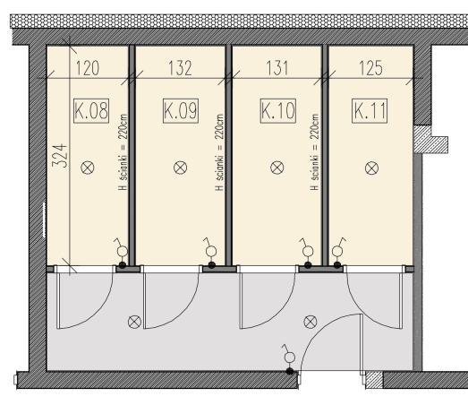
RZUT POMIESZCZEŃ
